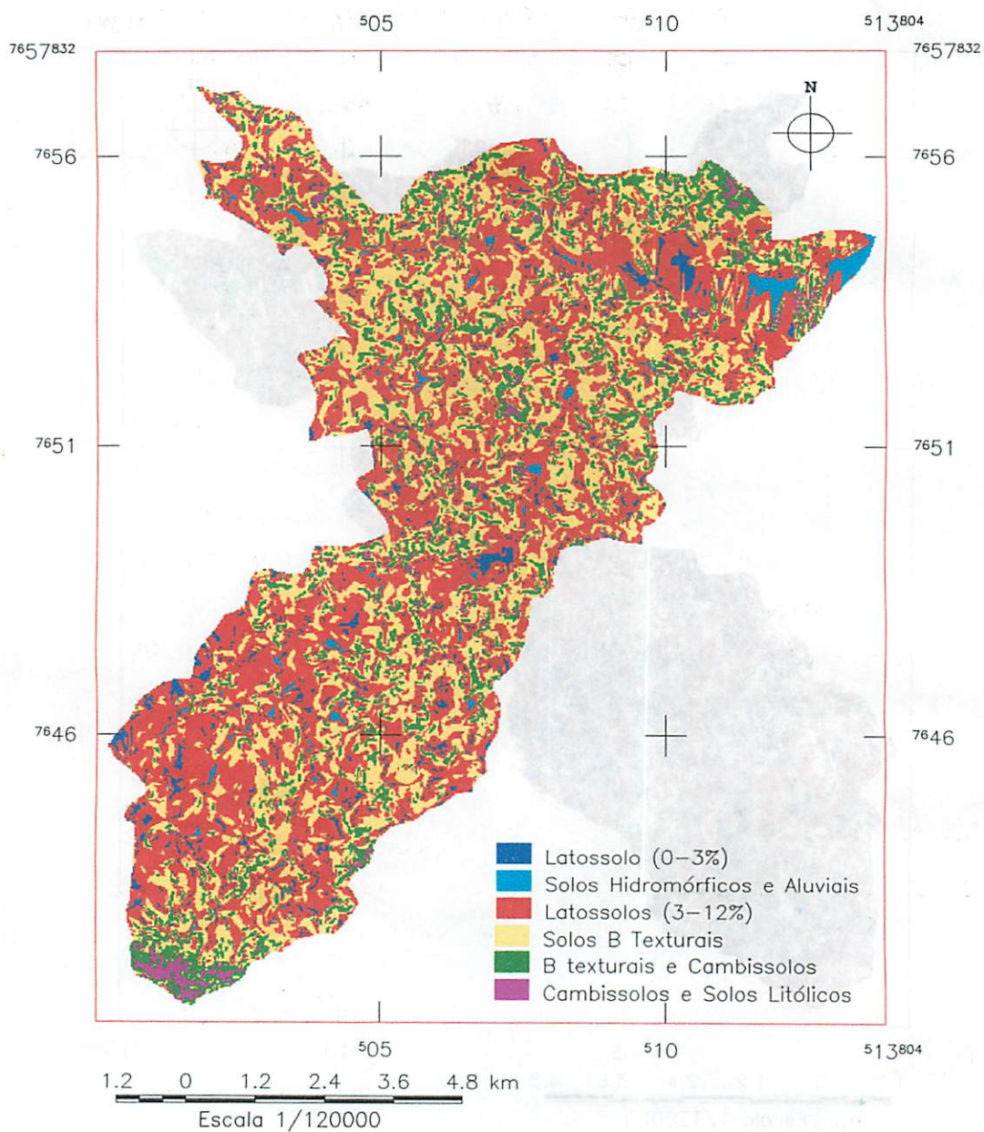
FIGURA 6 Mapa das classes de solos da sub-bacia do Ribeirão Santa Cruz, Lavras, MG.
