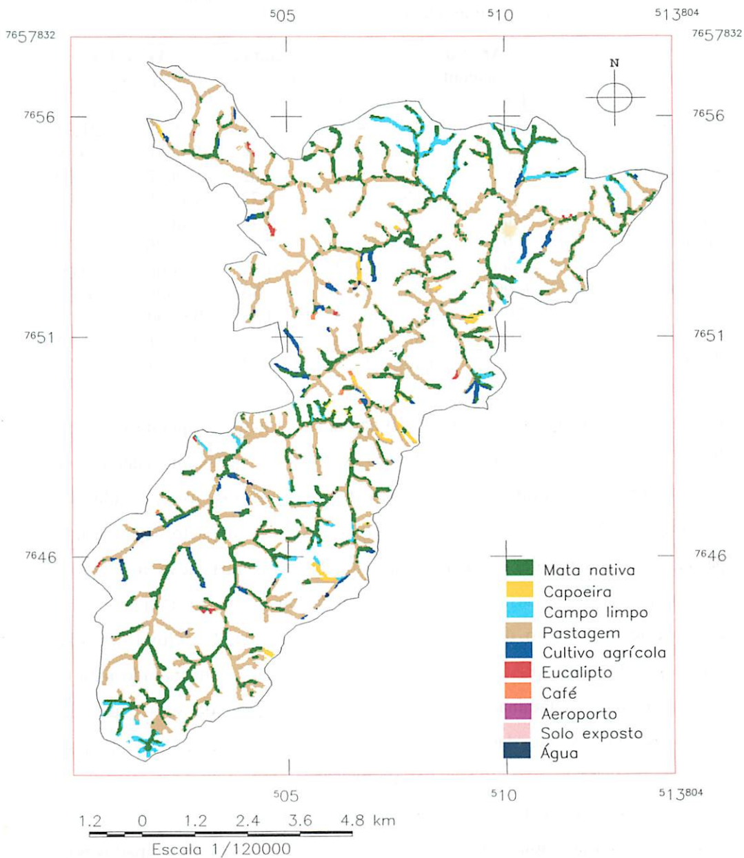
FIGURA 10 Mapa de uso da terra nas áreas de preservação permanente da sub-bacia do Ribeirão Santa Cruz, Lavras, MG.
