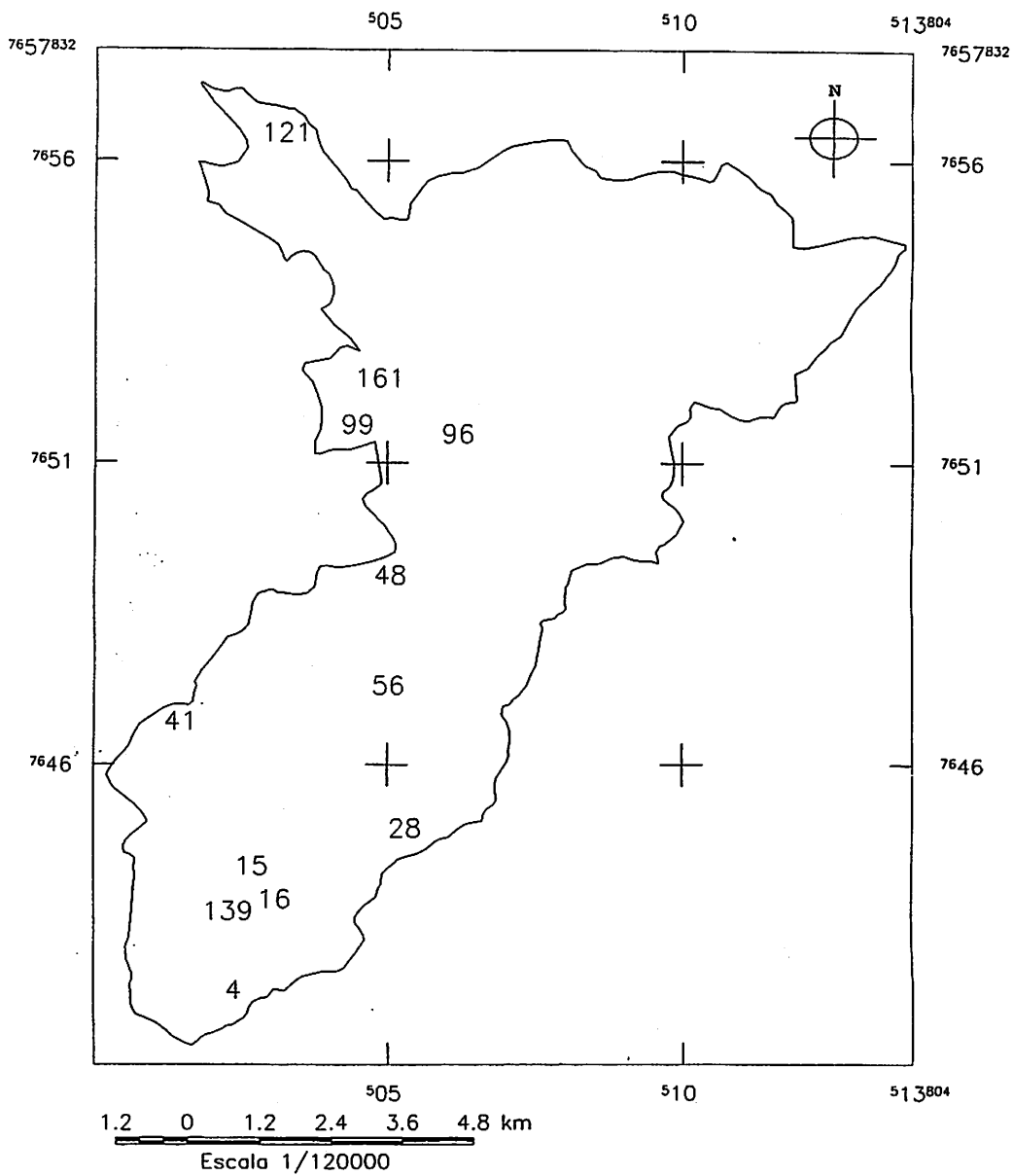
FIGURA 16 Mapa da localização das nascentes amostradas na sub-bacia do Ribeirão Santa Cruz, Lavras, MG.
