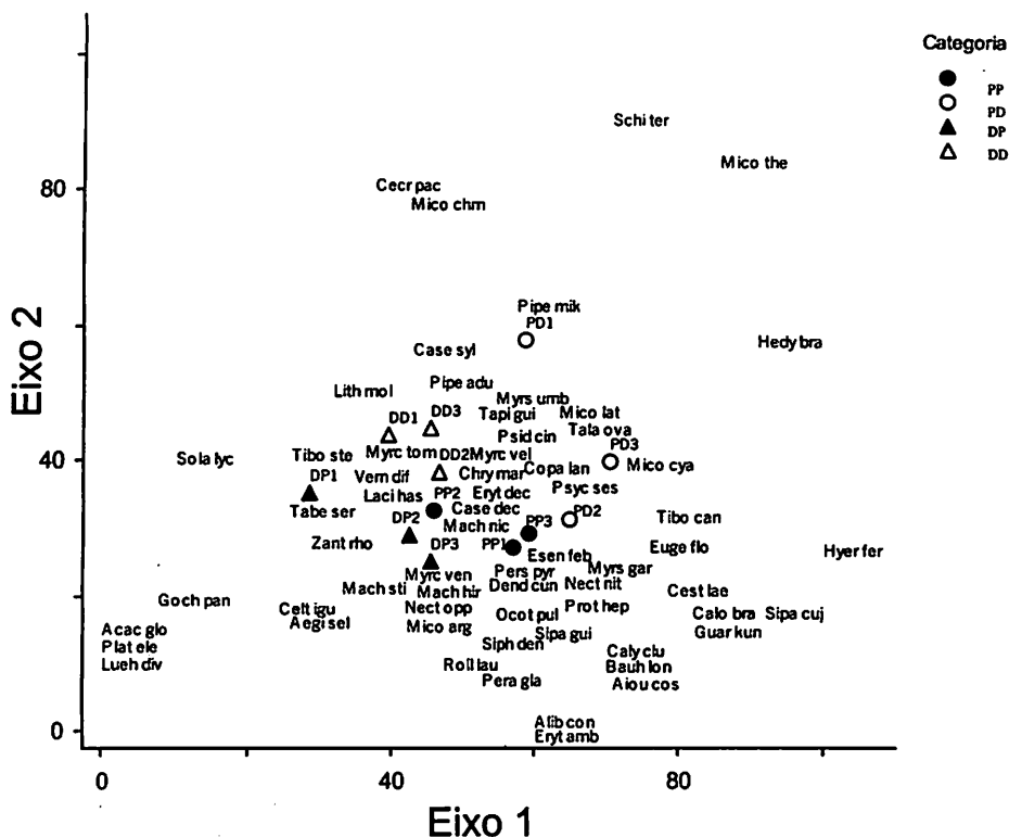
FIGURA 21 Diagrama de ordenação das espécies da regeneração natural dos doze fragmentos no entorno das nascentes da sub-bacia do Ribeirão Santa Cruz, Lavras, MG, produzido pela análise de correspondência retificada (DCA).
