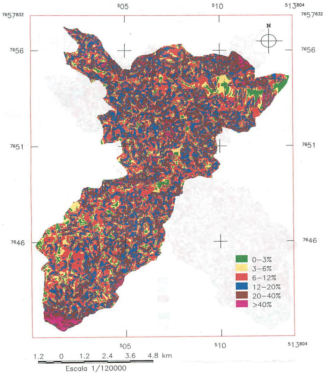
FIGURA 5 Mapa das classes de declividade da sub-bacia do Ribeirão Santa Cruz, Lavras, MG.
