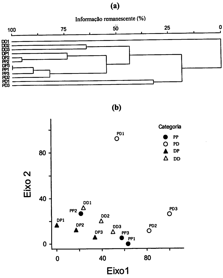
FIGURA 18 Análises multivariadas da composição da flora do estrato arbóreo e da regeneração natural dos doze fragmentos no entorno das nascentes da sub-bacia do Ribeirão Santa Cruz, Lavras, MG: (a) dendrograma de classificação, (b) diagrama de ordenação da análise de correspondência retificada (DCA).
