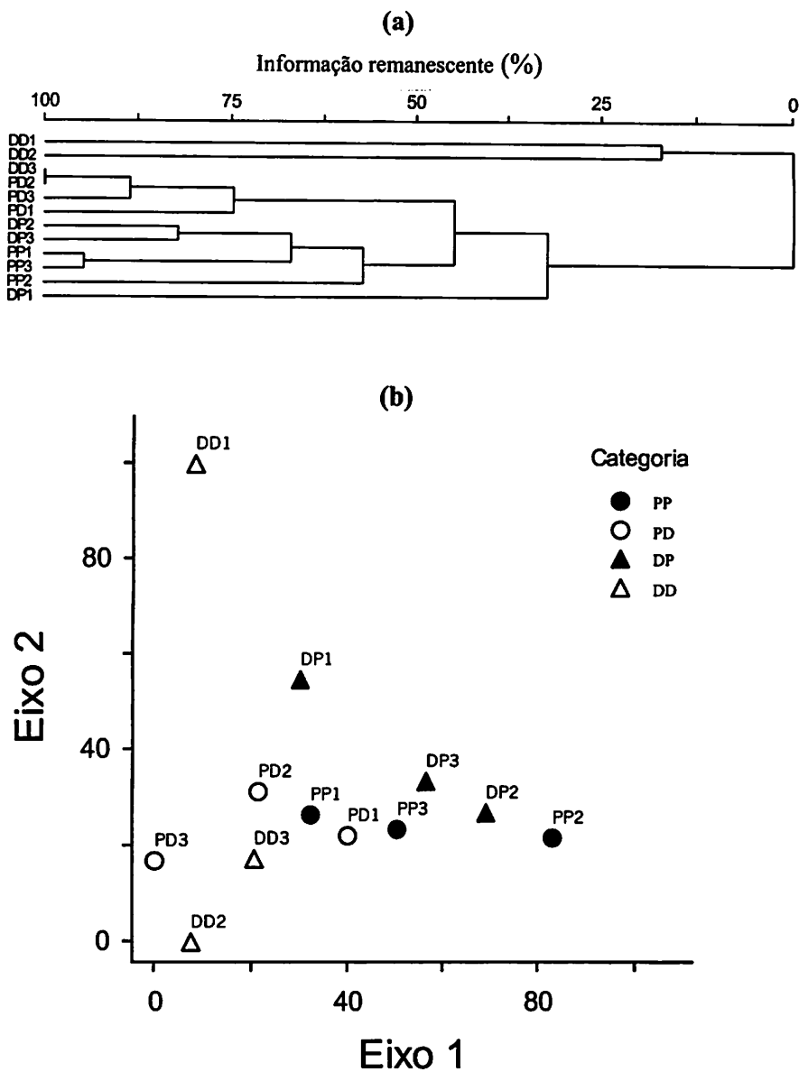
FIGURA 20 Análises multivariadas da composição da flora do estrato arbóreo dos doze fragmentos no entorno das nascentes da sub-bacia do Ribeirão Santa Cruz, Lavras, MG: (a) dendrograma de classificação, (b) diagrama de ordenação da análise de correspondência retificada (DCA).
