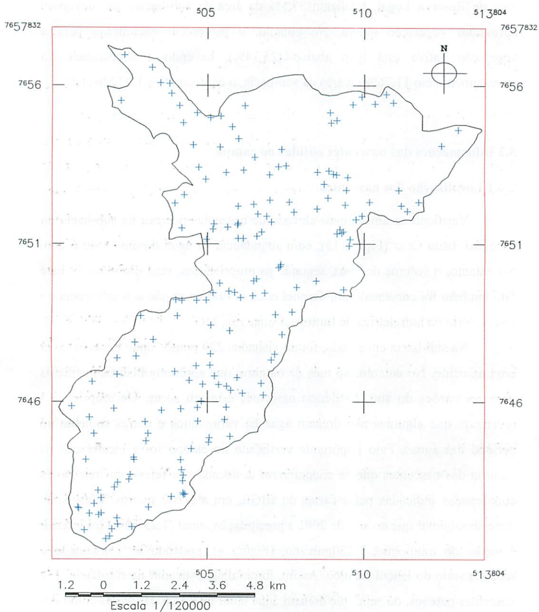
FIGURA 13 Localização das nascentes na sub-bacia do Ribeirão Santa Cruz, Lavras, MG.
