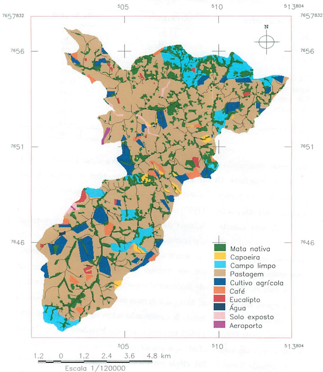
FIGURA 7 Mapa de uso da terra da sub-bacia do Ribeirão Santa Cruz, Lavras, MG.
