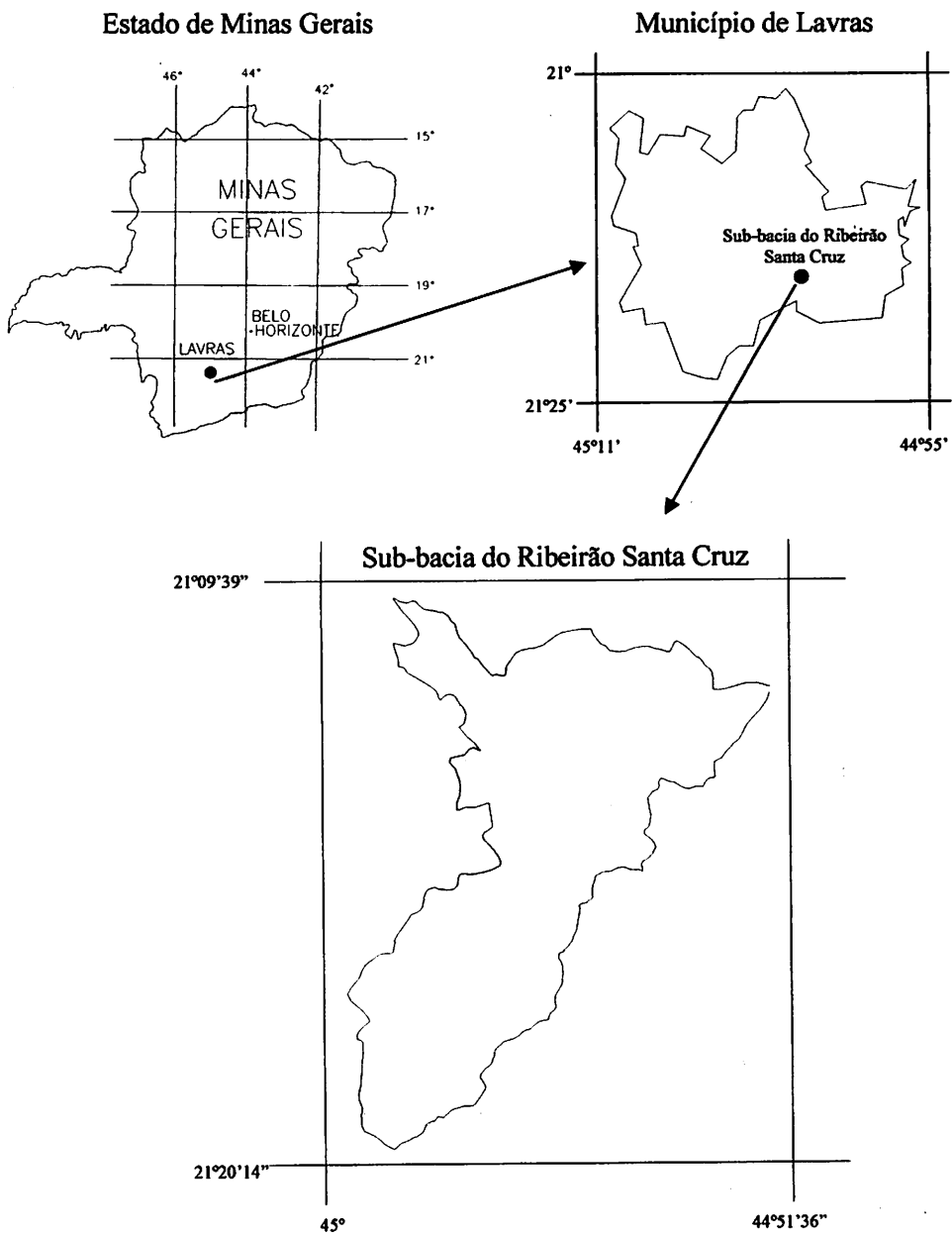
FIGURA 1 Localização da sub-bacia do Ribeirão Santa Cruz, Lavras, MG
