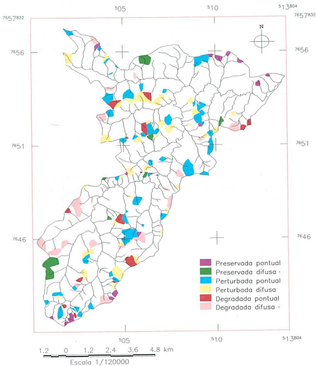
FIGURA 15 Mapa das áreas de recarga das nascentes da sub-bacia do Ribeirão Santa Cruz, Lavras, MG.
