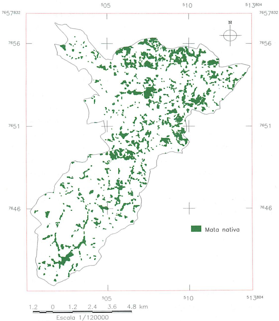
FIGURA 8 Mapa de mata nativa presente na sub-bacia do Ribeirão Santa Cruz, Lavras, MG.
