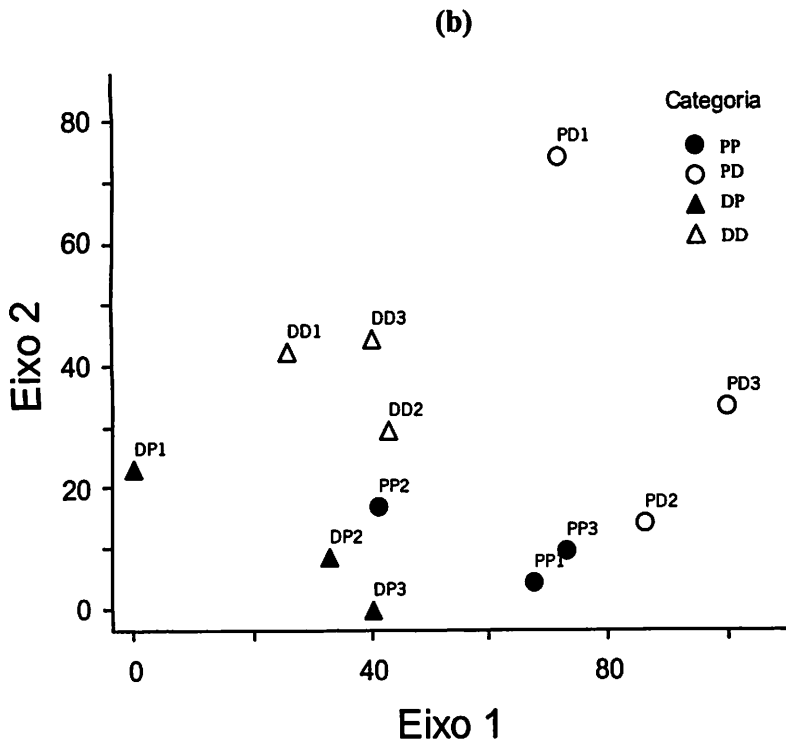
FIGURA 19 Análises multivariadas da composição da flora da regeneração natural dos doze fragmentos no entorno das nascentes da sub-bacia do Ribeirão Santa Cruz, Lavras, MG: (a) dendrograma de classificação, (b) diagrama de ordenação da análise de correspondência retificada (DCA).
