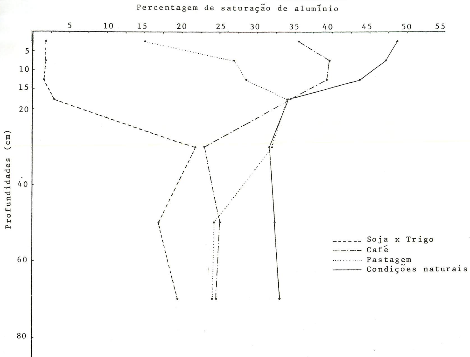
FIGURA 15 - Percentagem de saturação de alumínio em diferentes profundidades de um LV, nos diversos cultivos.
