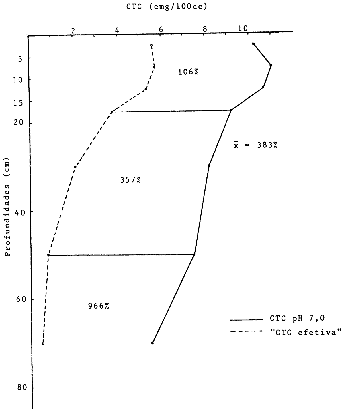
FIGURA 18 - Comparação entre " CTC efetiva" e CTC a pH 7,0 na rotação soja x trigo, em diferentes profundidades de um LV.
