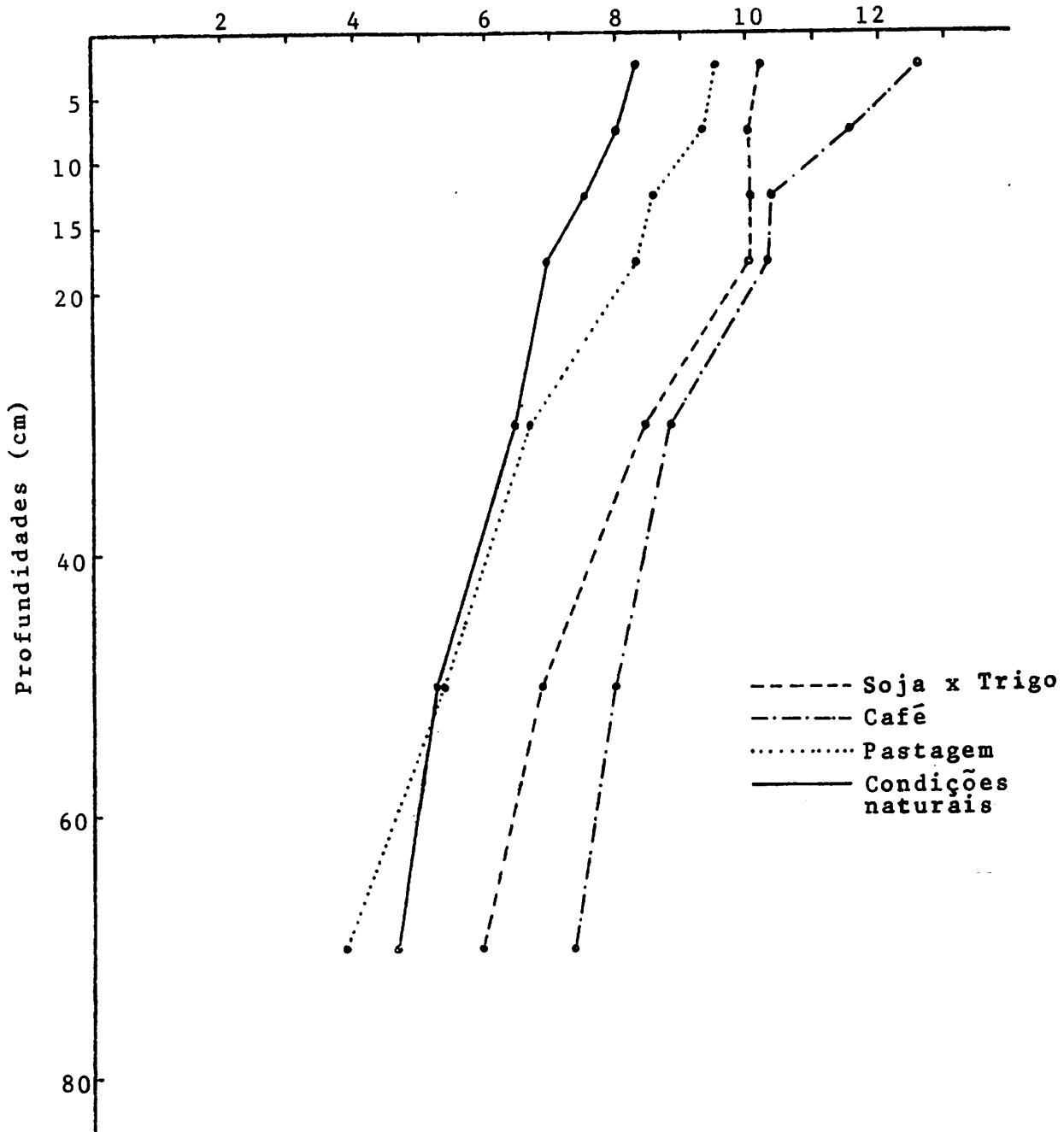
FIGURA 13 - Capacidade de troca de cations total do solo em diferentes profundidades de um LV, nos diversos cultivos.
