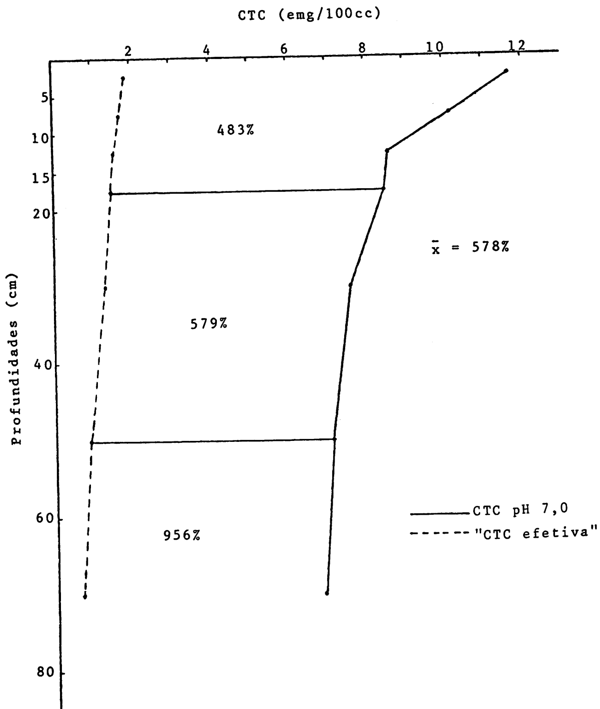
FIGURA 21 - Comparação entre "CTC efetiva" e CTC a pH 7,0 no café, em diferentes profundidades de um LV.
