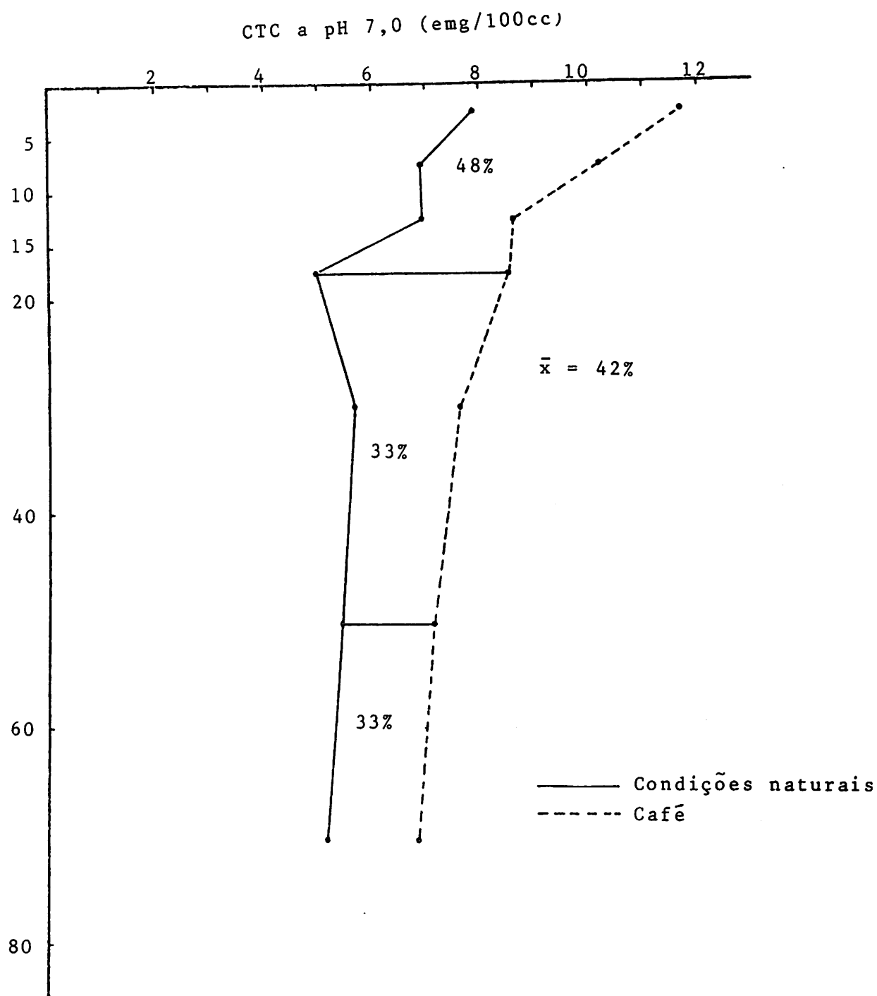
FIGURA 22 - Comparação entre CTC a pH 7,0 em condições naturais e CTC a pH 7,0 no café, em diferentes profundidades de um LV.
