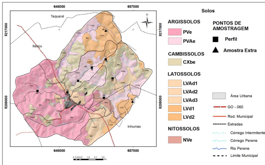
Figura 4. Mapa de solos da bacia hidrográfica do alto rio Meia Ponte.
