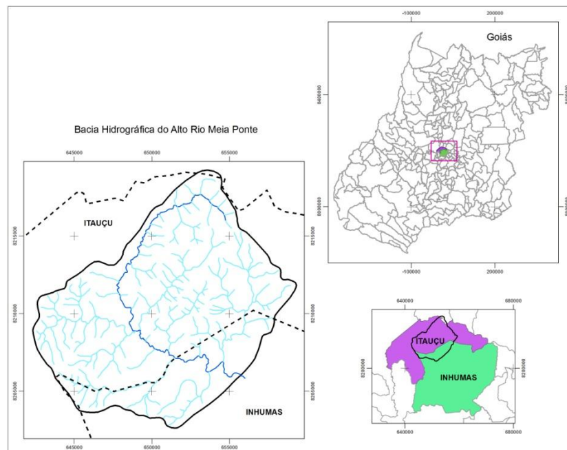
Figura 1. Bacia hidrográfica do alto Meia Ponte, GO
