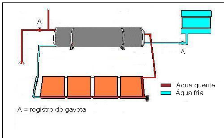
Figura 4.1 – Sistema de aquecimento fase I
