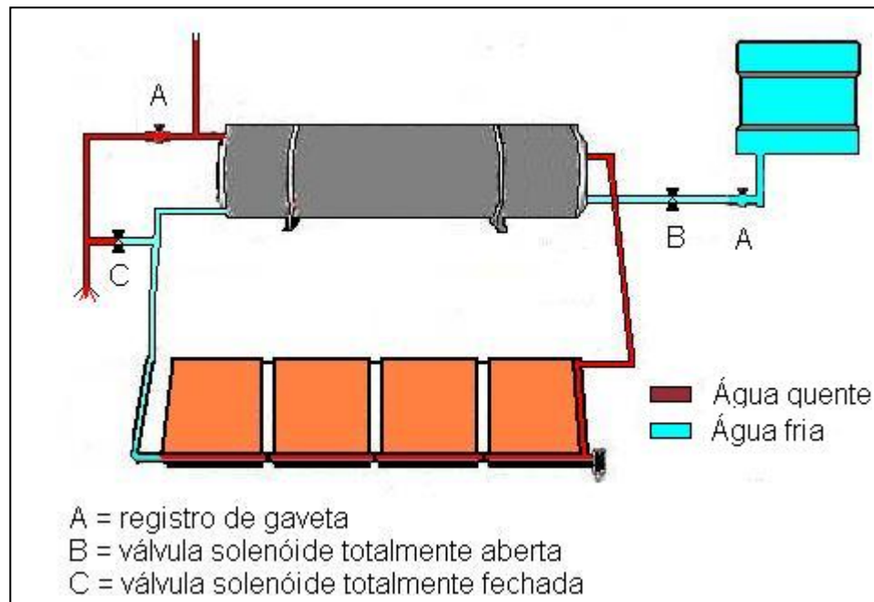
Figura 4.3 – Sistema de aquecimento fase II de dia
