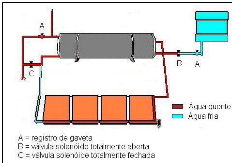
Figura 4.2 – Sistema de aquecimento fase II à noite
