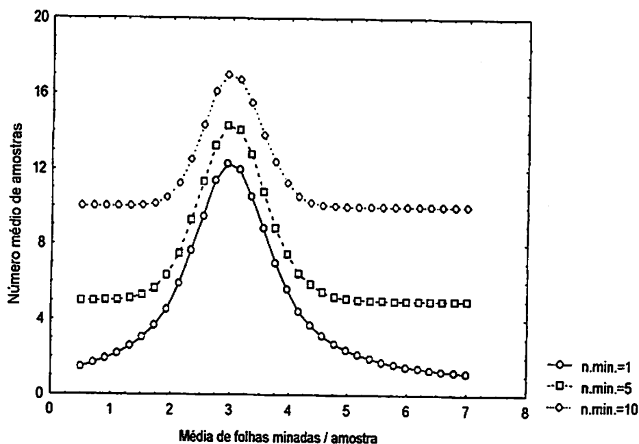
FIGURA 11 Número médio de amostras do plano de amostragem seqüencial, para avaliar o número de folhas minadas por P. coffeella , na região dos terços médio e superior da planta, comparando o efeito do número mínimo de amostras (n máximo = 20).
