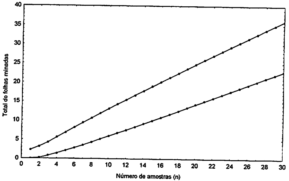
FIGURA 3 Linhas de decisão, para amostragem seqüencial de folhas minadas por P. coffeella , no terço médio de cafeeiros, na região de Lavras, MG.
