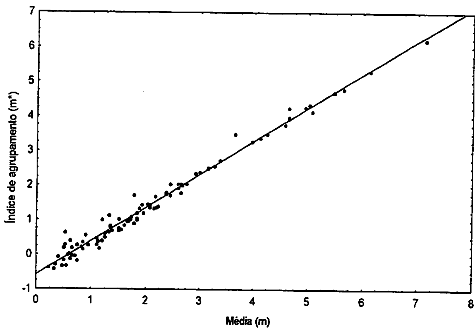
FIGURA 2 Relação entre o índice de agrupamento ( m^* ) e a média ( m ), a partir do número de folhas minadas por P. coffeella , na região do terço médio e superior da planta. Modelo de Lloyd: m^* = -0,574 + 0,965m , ( R^2 = 0,98 , P < 0,001 ).
