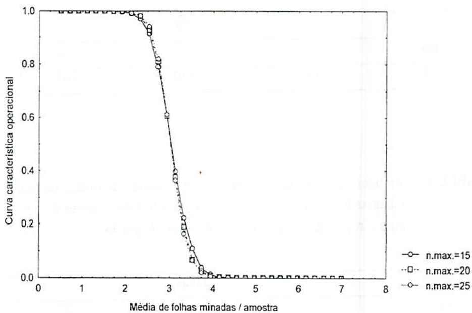
FIGURA 10 Curva característica operacional do plano de amostragem seqüencial, para avaliar o número de folhas minadas por P. coffeella , na região dos terços médio e superior da planta, comparando o efeito do número máximo de amostras ( n mínimo = 5).
