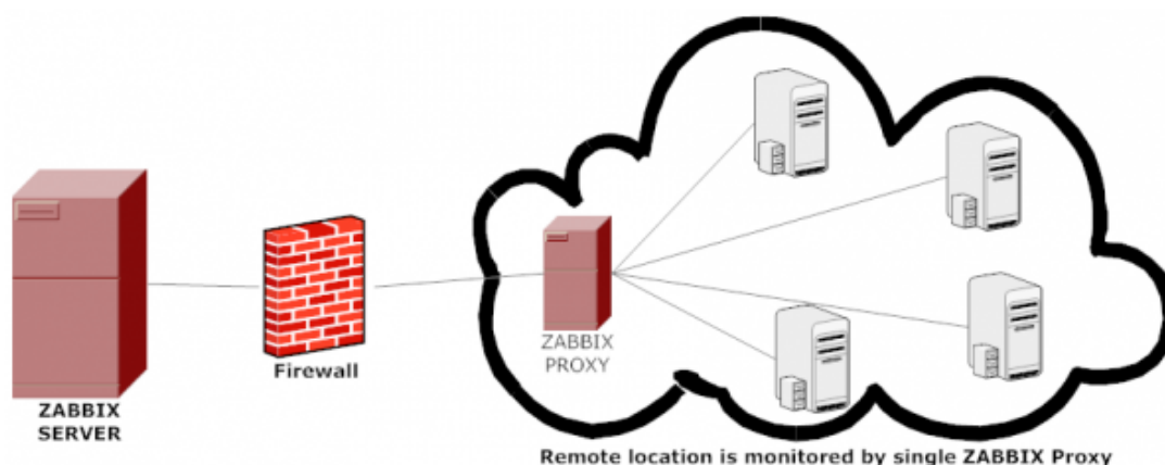
Figura 4.6 – Topologia genérica, como exemplo de uso do Zabbix Proxy
