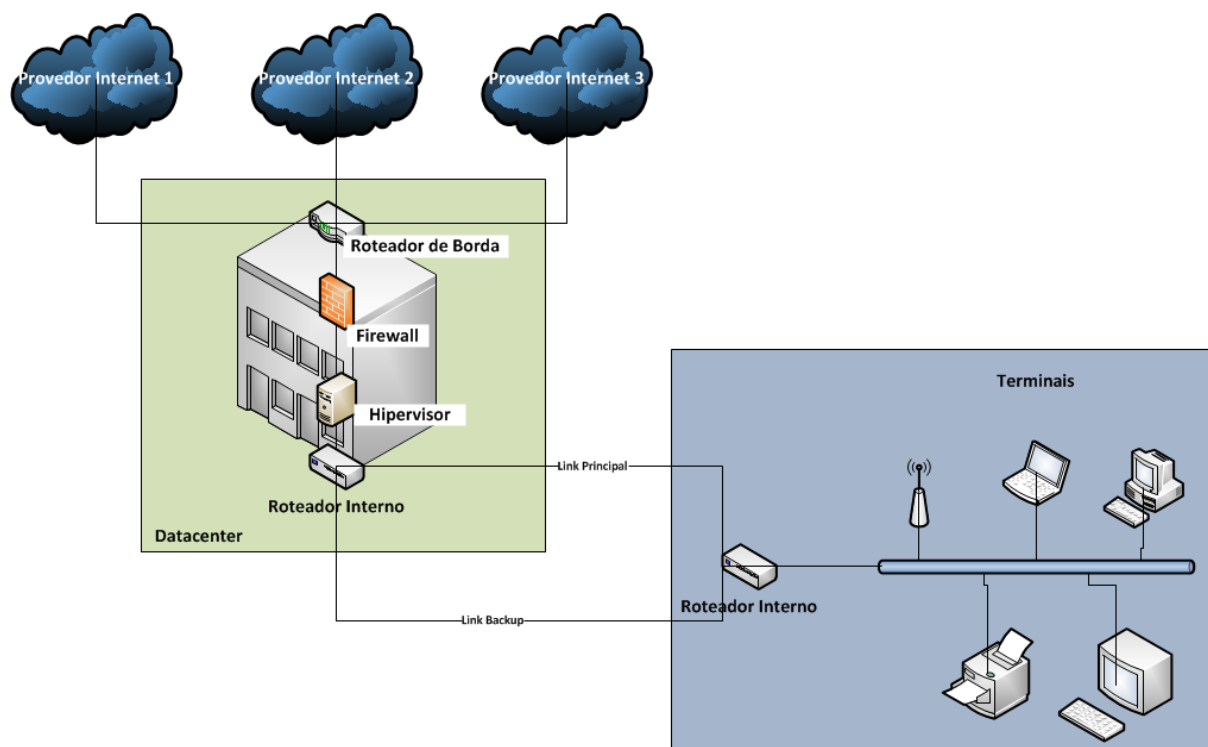
Figura 4.1 – Estrutura básica da Rede monitorada.
