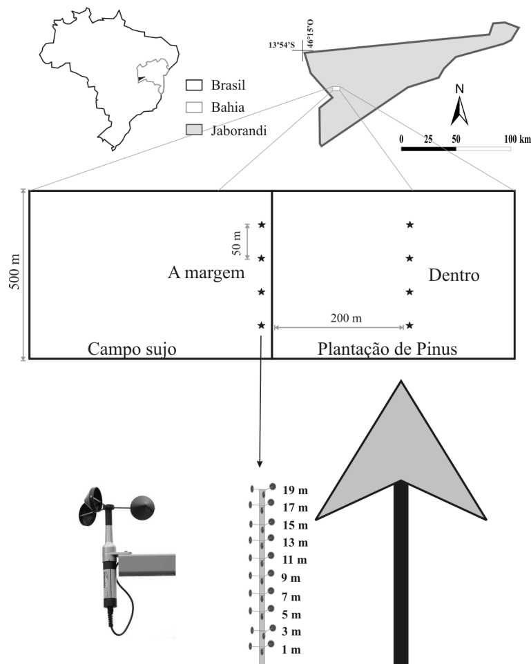
Figura 1 – Localização da área de estudo e disposição das torres com os anemômetros.
