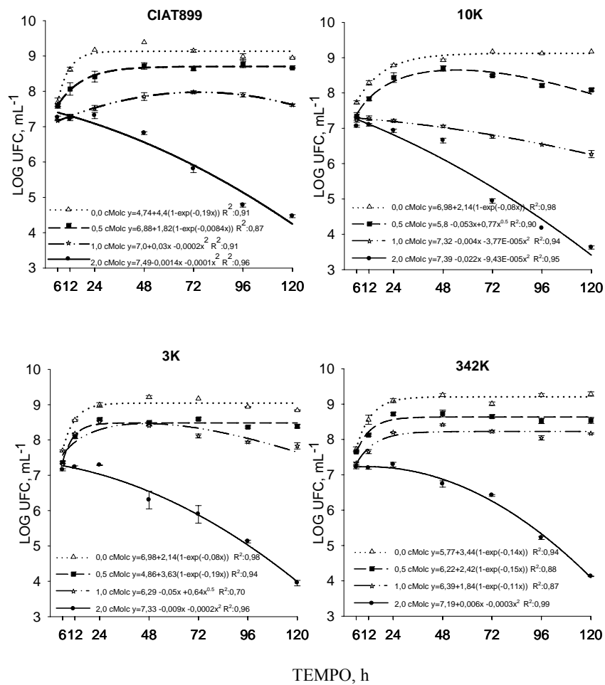
Figura 7. Crescimento das estirpes CIAT899, 10K, 3K e 342K em meio líquido em função das diferentes concentrações de Al 3+ no meio de cultivo.
