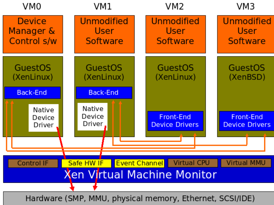
Figura 2.3: Para-Virtualização (XEN, 2005)
