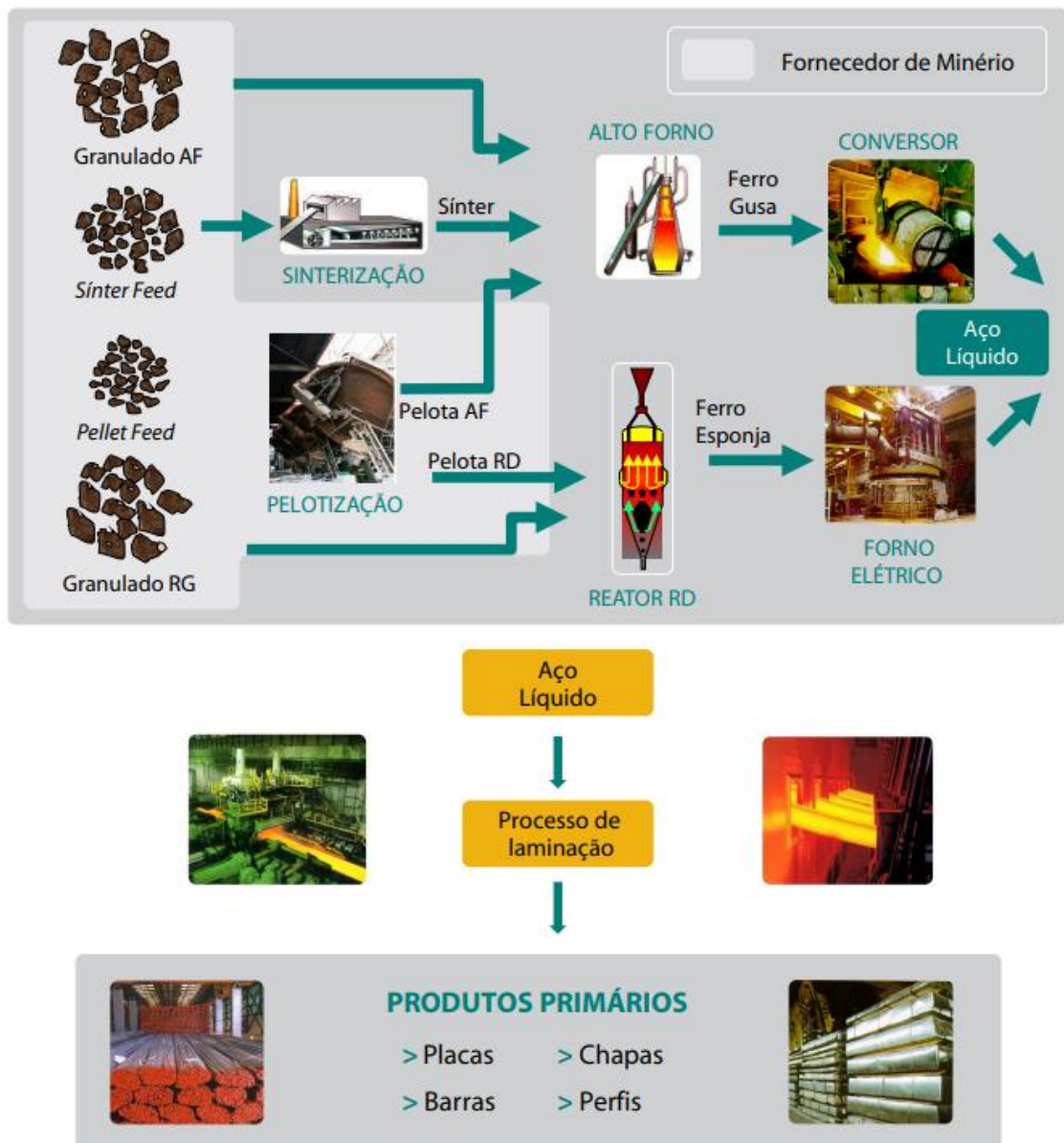
Figura 6 – Etapas Siderúrgicas para a produção do Aço
