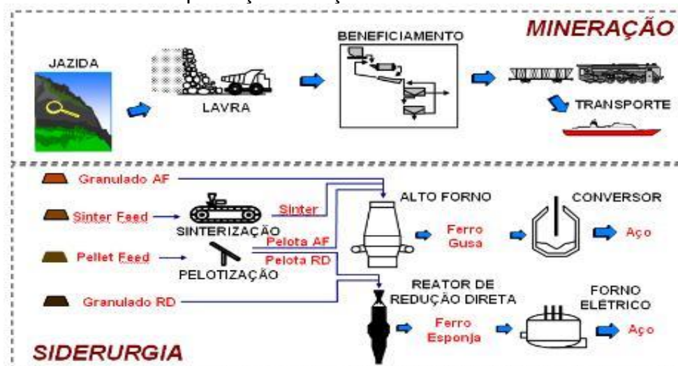
Figura 1 – Etapas do Processo de beneficiamento do Ferro e da produção do Aço
