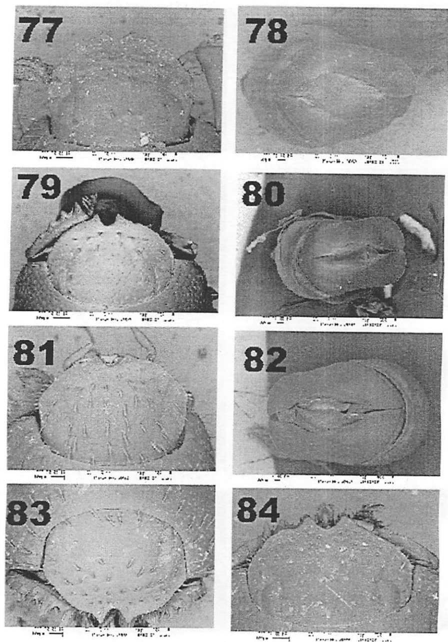
FIGURES 77-84. Dorsal view of head and paramera. 77-78. Trichillum ballerioi ; 79-80. T. belloi ; 81-82. T. bellorum ; 83. T. borrei ; 84. T. canhedoae .
