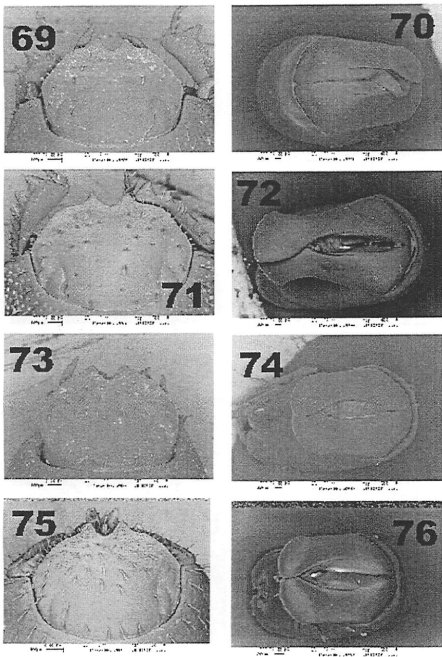
FIGURES 69-76. Dorsal view of head and paramera. 69-70. Trichillum depilatum ; 71-72. T. halffteri ; 73-74. T. andersoni ; 75-76. T. arriagadai .
