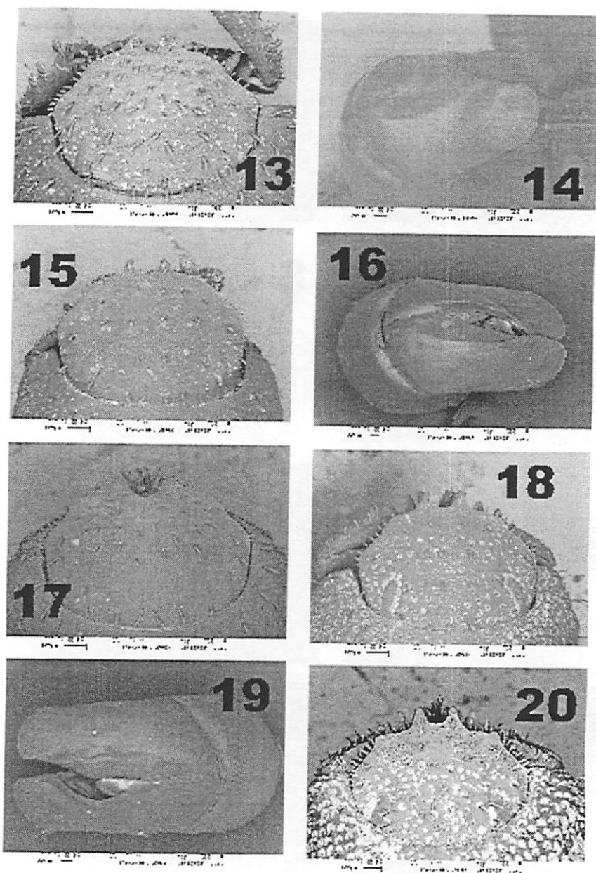
FIGURES 13-20. Dorsal view of head and paramera. 13-14. Besourenga guimaraesrosai ; 15-16. B. michelleae ; 17. B. renaudpauliani ; 18-19. B. sergioidei ; 20. B. sprecherae .
