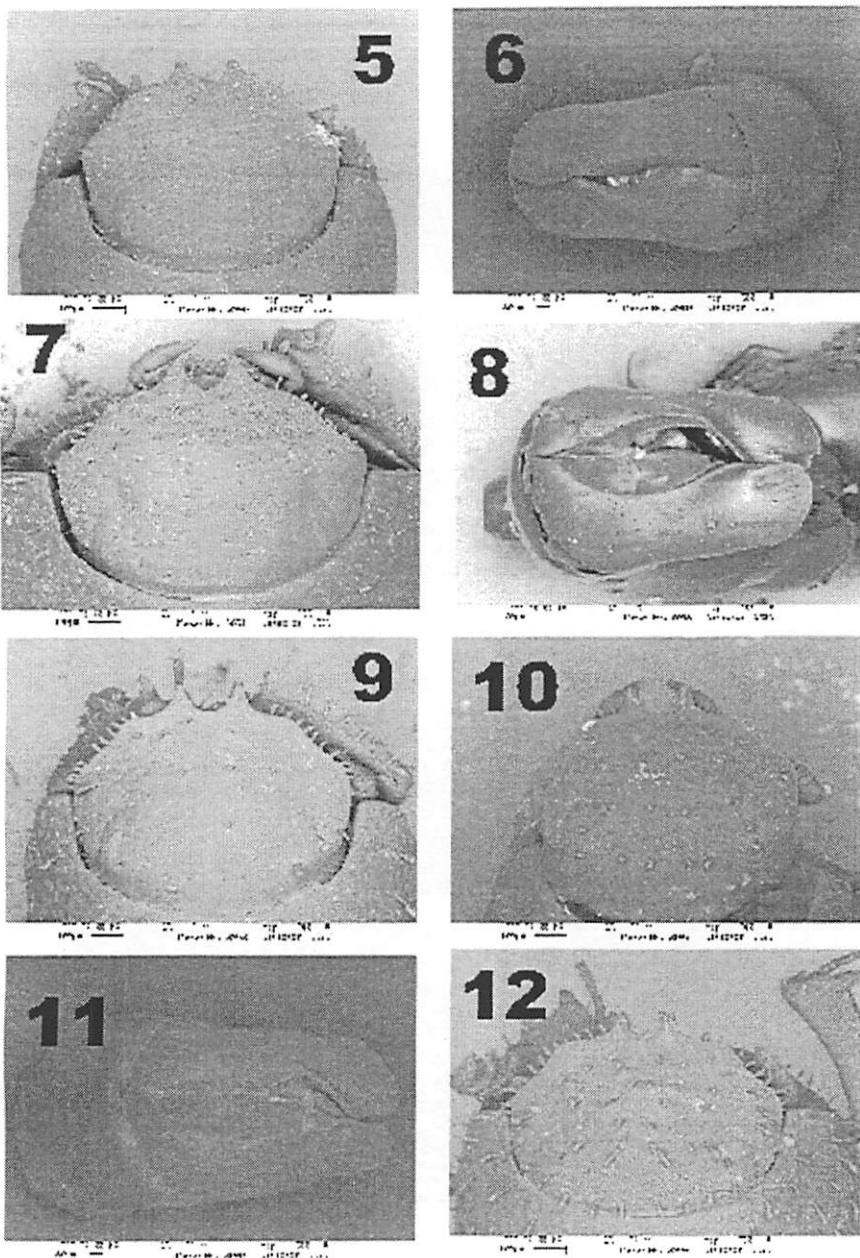
FIGURES 5-12. Dorsal view of head and paramera. 5-6. Besourengea minutus ; 7-8. B. vejvodskyi ; 9. B. bachmanni ; 10-11. B. brucei ; 12. B. campaneri .
