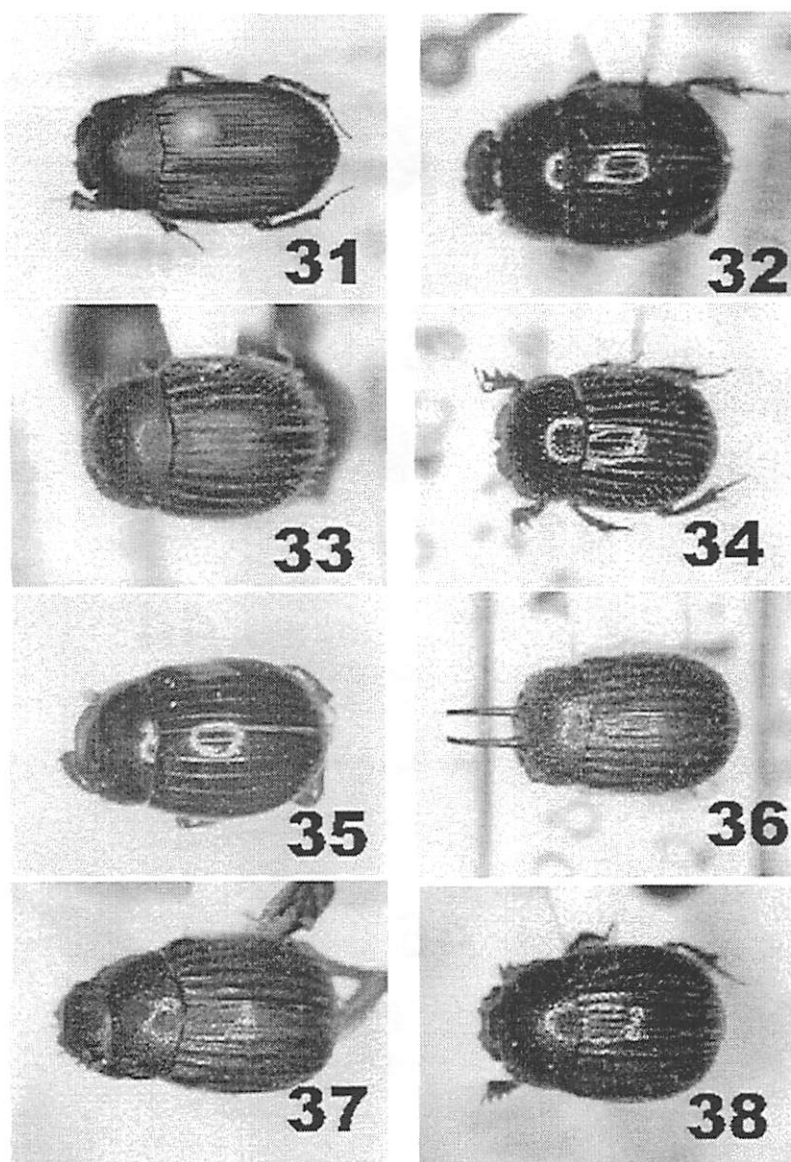
FIGURES 31-38. Dorsal view. 31. Pedaridium hirsutum ; 32. Trichillum ( Trichillum ) heydeni ; 33. T. ( Paratrichillum ) pauliani ; 34. Eutrichillum onorei ; 35. Silvia unica ; 36-37. Pereiraidium almeidai (36. \Gamma ; 37. E ); 38. Onoreidium ohausi .
