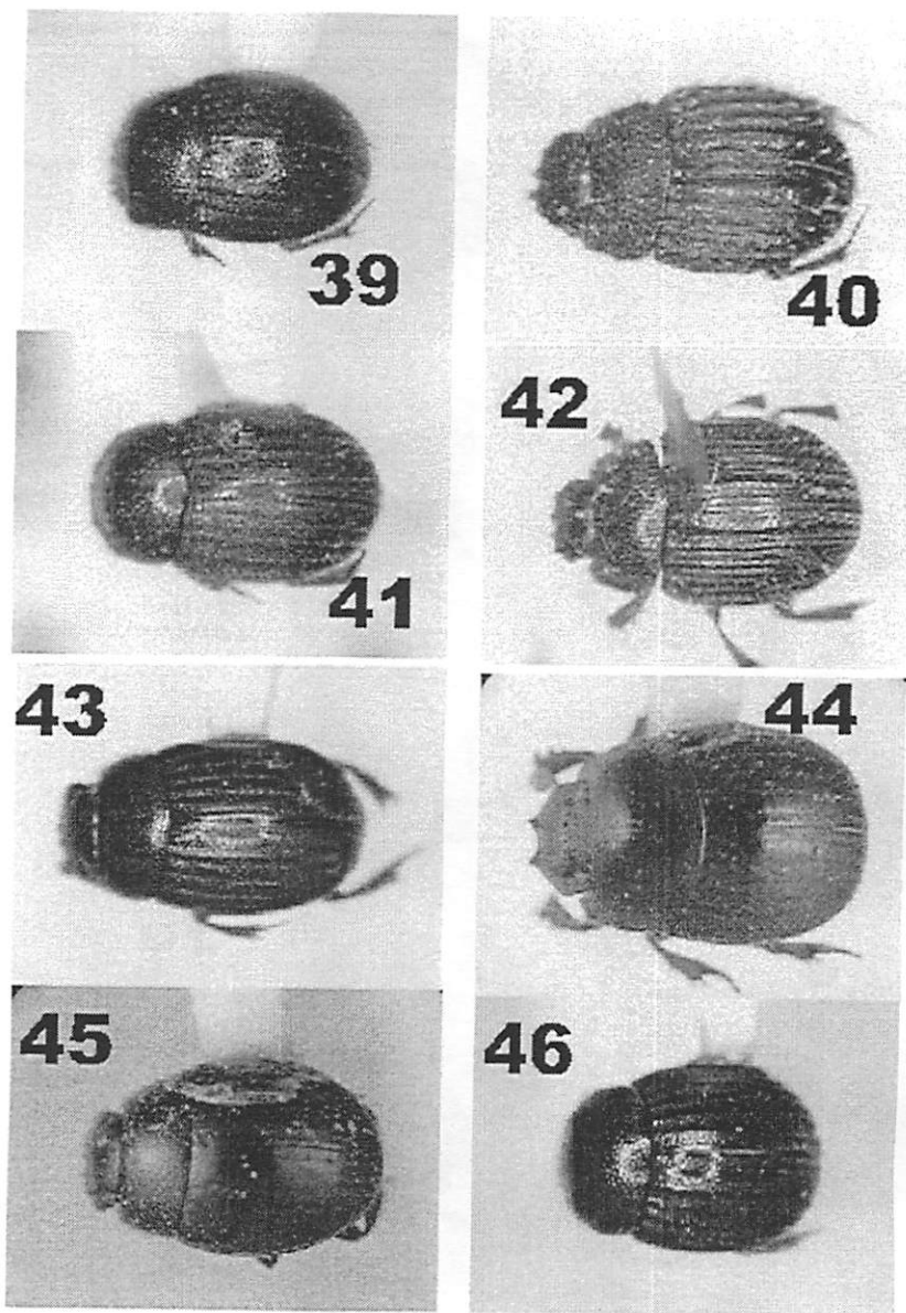
FIGURES 39-46. Dorsal view. 39. Trichillidium quadridens ; 40. Horridotrichillum horacioi ; 41. Besourengea michelleae ; 42. B. sprecherae ; 43. Bradypodidium bustamantei ; 44. Howdenidium bottimeri ; 45. Youngidium brevisetosum ; 46. Boreotrichillum pilosum .
