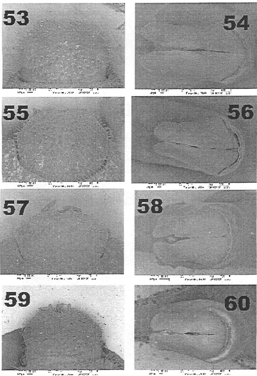
FIGURES 53-60. Dorsal view of head and paramera. 53-54. Genieridium bordoni ; 55-56. G. paranense ; 57-58. G. zanunciorum ; 59-60. G. cryptops .
