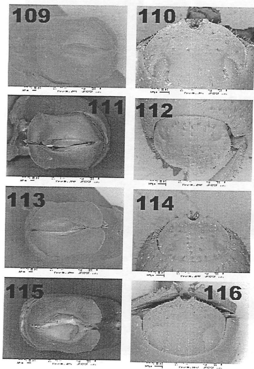
FIGURES 109-116. Dorsal view of head and paramera. 109. Trichillum moacyri ; 110-111. T. paschoali ; 112-113. T. peckorum ; 114-115. T. schefflerorum ; 116. T. schoerederi .
