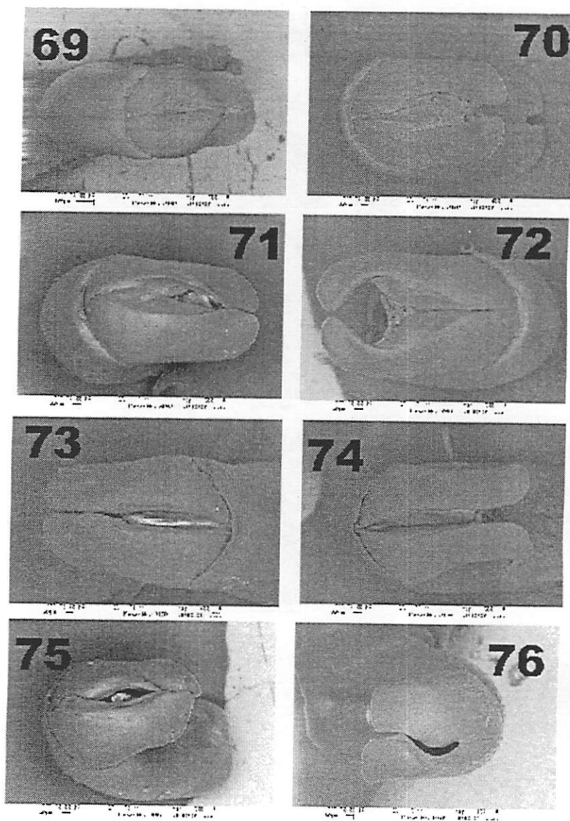
FIGURES 69-76. Dorsal view of paramera. 69. Pedaridium hirsutum ; 70. Trichillum (Paratrichillum) pauliani ; 71. Besourengea michelleae ; 72. Silvia unica ; 73. Pereiraidium almeidai ; 74. Onoreidium ohausi ; 75. Horridotrichillum horacioi ; 76. Besourengea ubirajarai .
