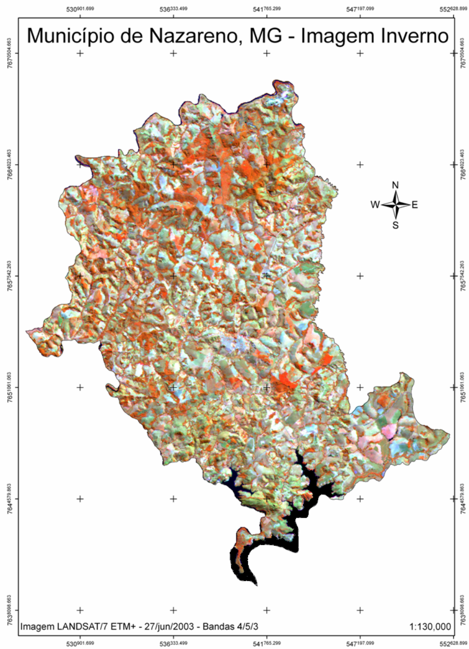
FIGURA 4 - Imagem LANDSAT/7 - ETM + - Município de Nazareno, data de passagem 27 de junho de 2003 (imagem inverno).
