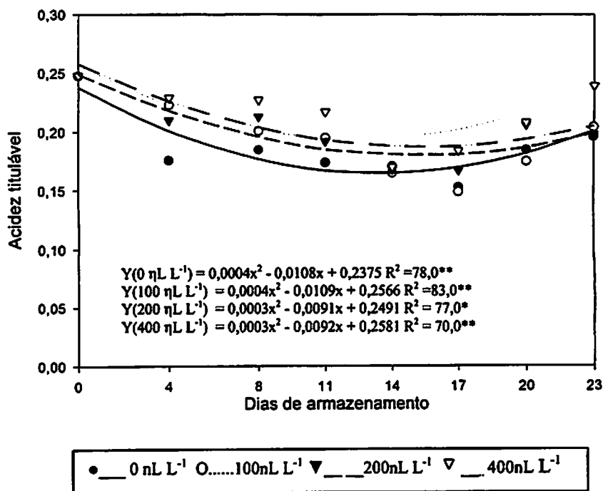
FIGURA 6 Acidez titulável (% ácido málico) de sapotis tratados com diferentes concentrações (0, 100, 200, 400ηL L -1 ) de 1-MCP e armazenados, sob atmosfera modificada, à temperatura de 25 ± 2°C e 70 ± 5% UR.
