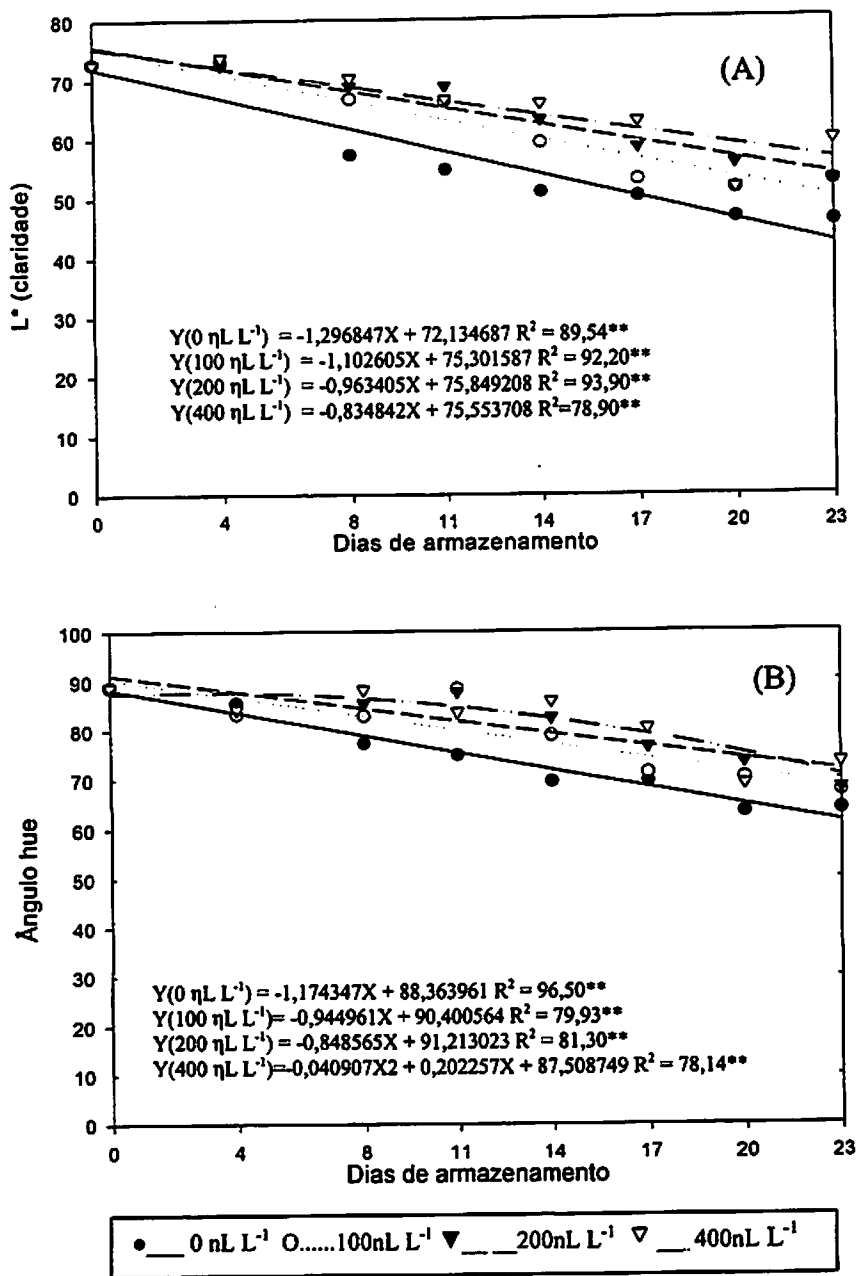
FIGURA 4 L* (claridade) (A) e ângulo hue (B) da cor da polpa de saptis tratados com diferentes concentrações (0, 100, 200, 400ηL L -1 ) de 1-MCP e armazenados, sob atmosfera modificada, à temperatura de 25 ± 2°C e 70 ± 5% UR.
