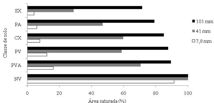
Figura 8 Áreas saturadas durante as precipitações diárias, relativas a cada classe de solo
