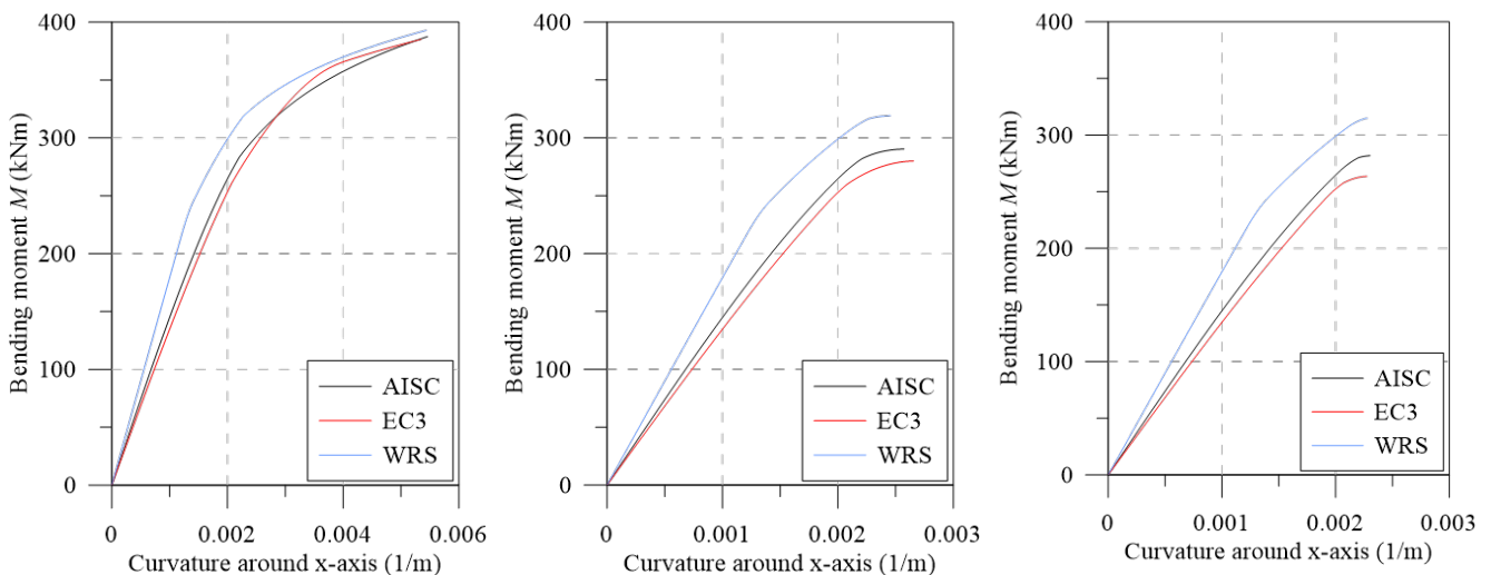
(d) For N = 8000 kN and \gamma = 0
