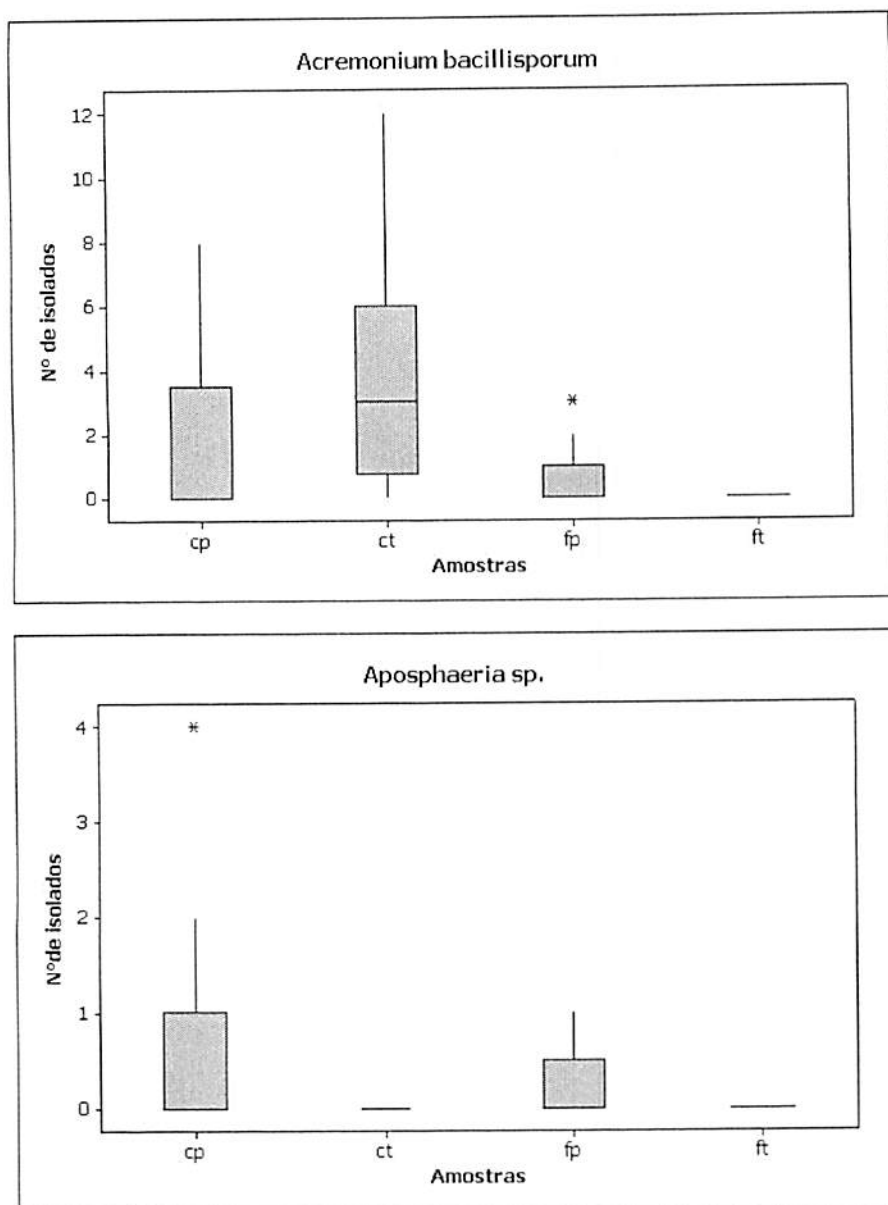
FIGURA 5 Box plot mostrando a variação no número de isolados recuperados em cada tecido para alguns fungos mais freqüentemente isolados (continua...).
