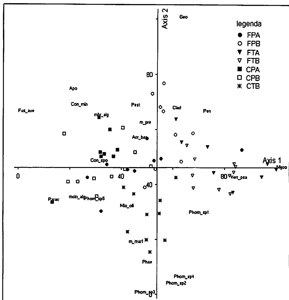
FIGURA 4 Gráfico gerado pela análise estatística multivariada DCA mostrando as semelhanças entre amostras e espécies de fungos endófitos. FP, CP - folhas e caules de P. perrottettii ; FT e CT - folhas e caules de T. guianensis ; A - amostras da primeira coleta; B - amostras da segunda coleta.
