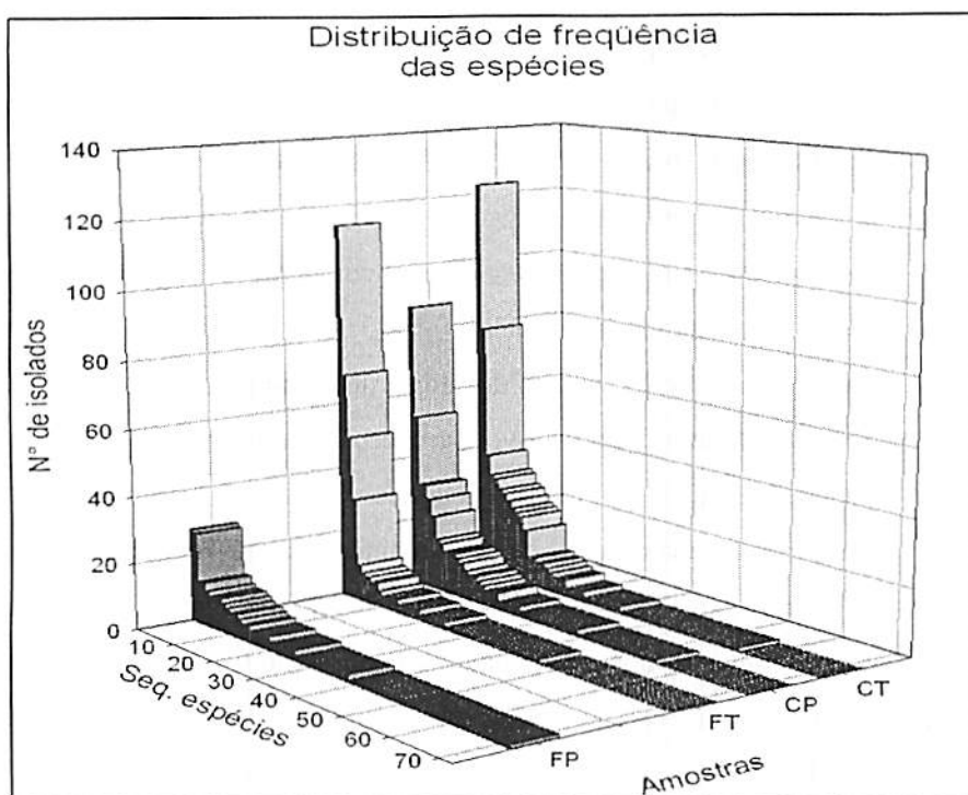
FIGURA 3 Distribuição de freqüência de isolamento das espécies de fungos endófitos nos quatro tecidos amostrados. FP, CP - folhas e caules de P. perrottettii ; FT e CT - folhas e caules de T. guianensis .
