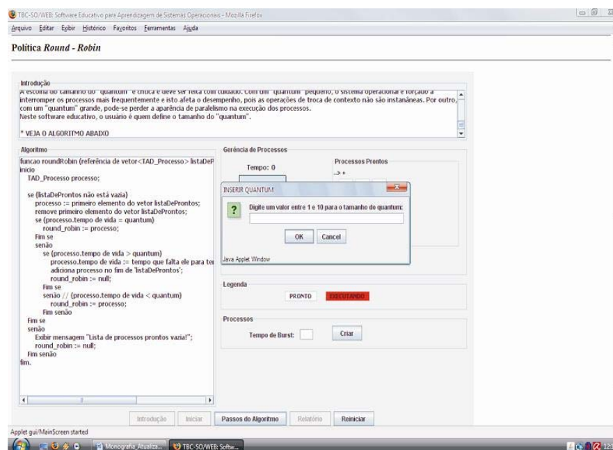
Figura 7-20 – Janela “Inserir Quantum” na Política Round-Robin
