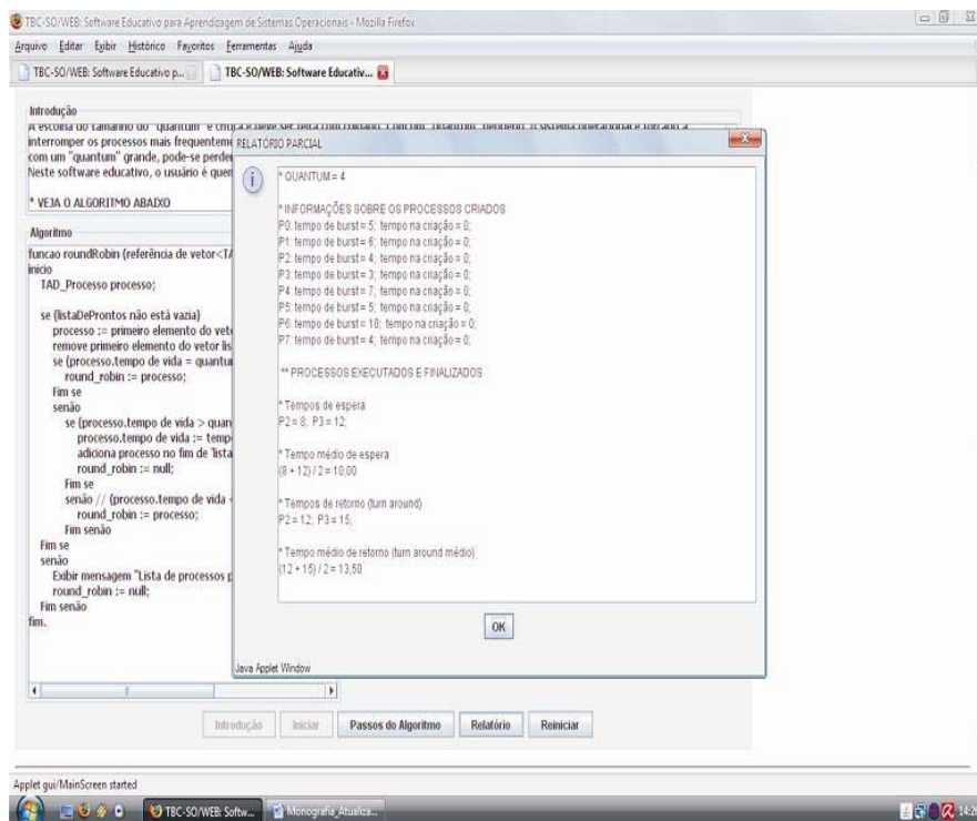
Figura 7-18 – Tela de Execução da Política de Gerência de Processos Round-Robin com Janela de Relatório
