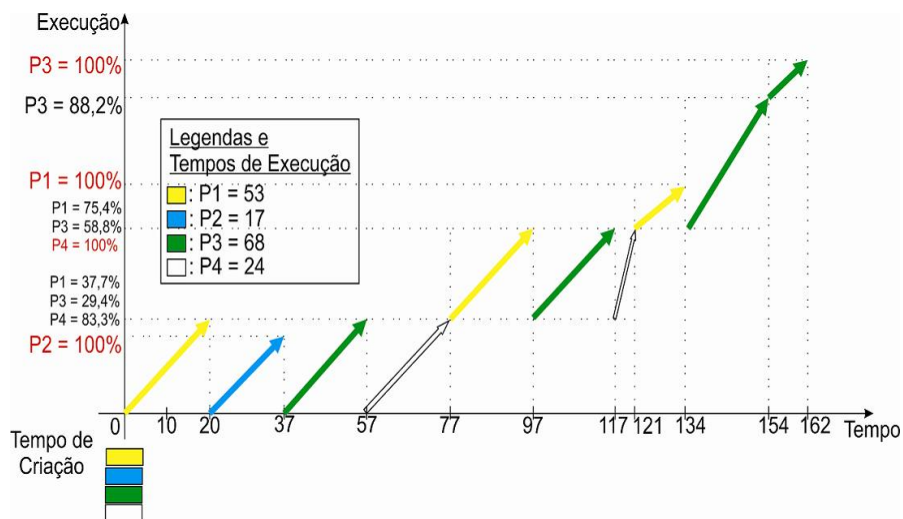
Figura 4-7 – Exemplo de Uso da Política Round-Robin
