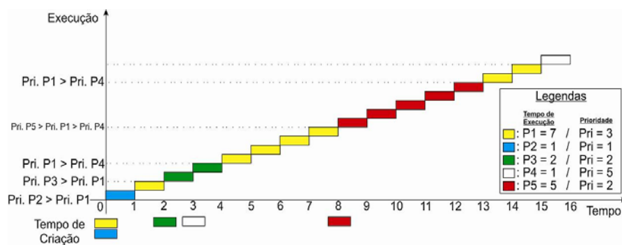
Figura 4-6 – Exemplo de Uso da Política Por Prioridade Preemptiva
