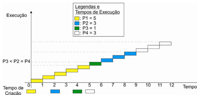
Figura 4-2 – Exemplo de Uso da Política SJF
