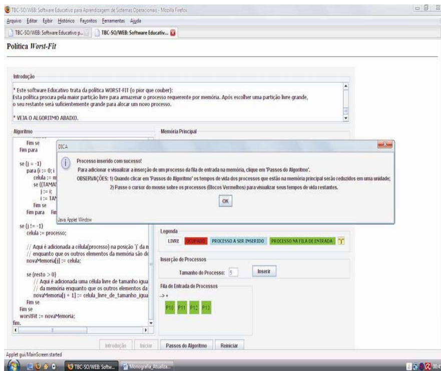
Figura 7-12 – Tela com Mensagem de Sucesso após Inserir um Processo
