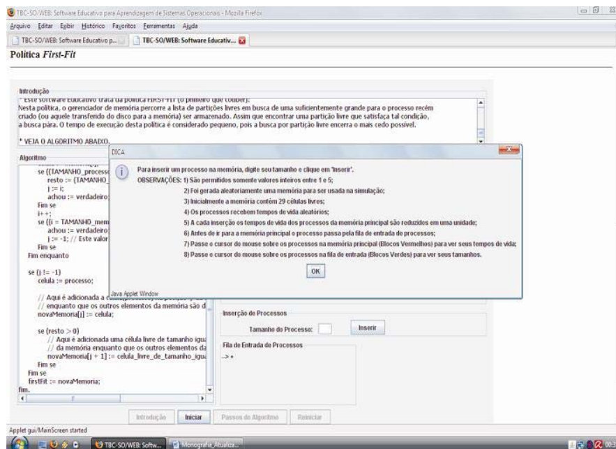
Figura 7-10 – Tela da Política de Gerência de Memória First-Fit
