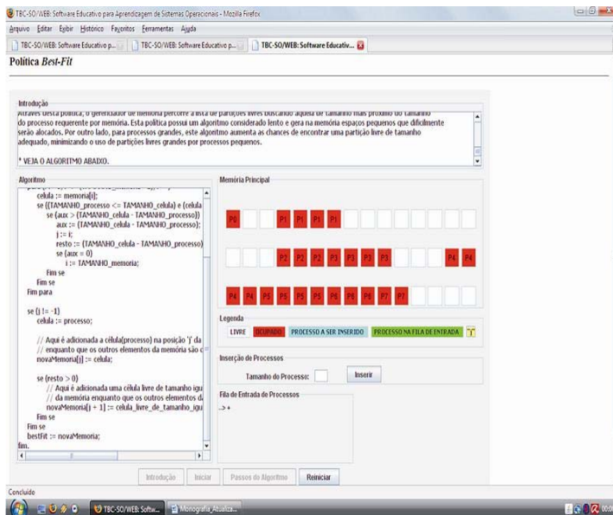
Figura 7-6 – Tela Inicial da Política de Gerência de Memória Best-Fit
