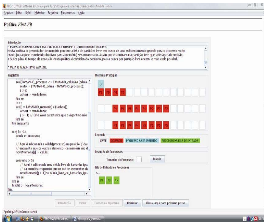
Figura 7-9 – Tela de Execução da Política First-Fit
