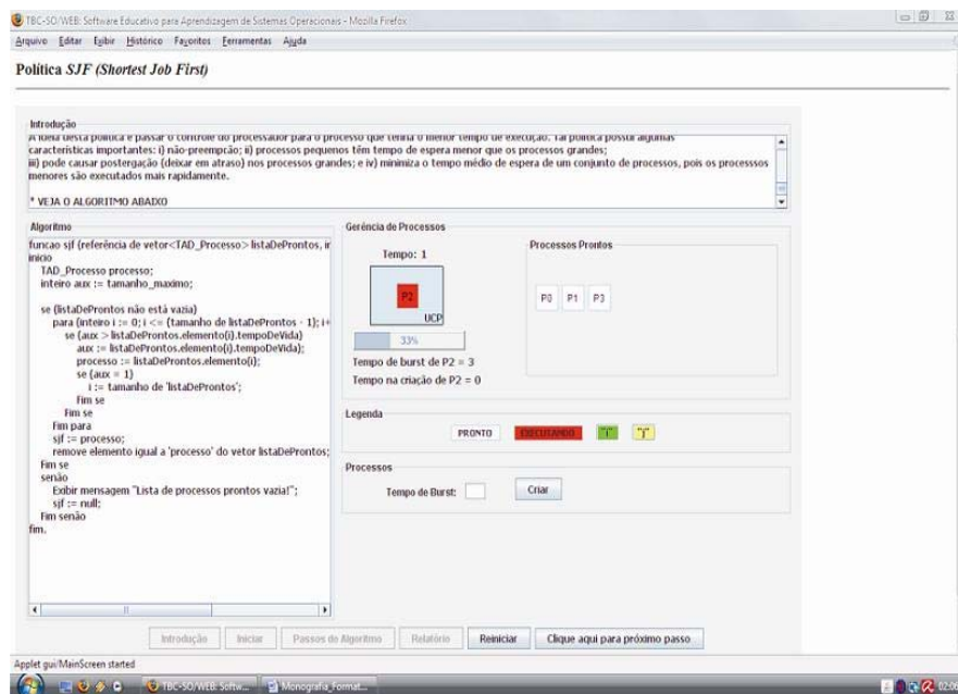
Figura 7-19 – Tela da Política SJF Executando um Processo
