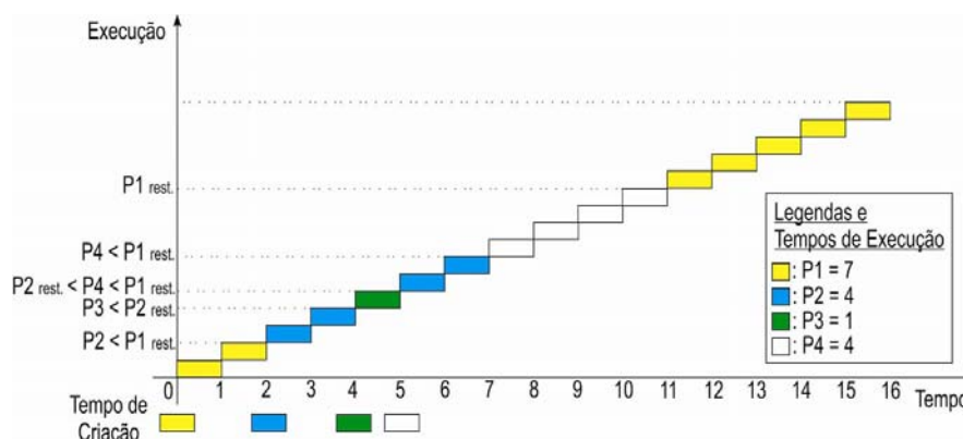
Figura 4-3 – Exemplo de Uso da Política SRTF
