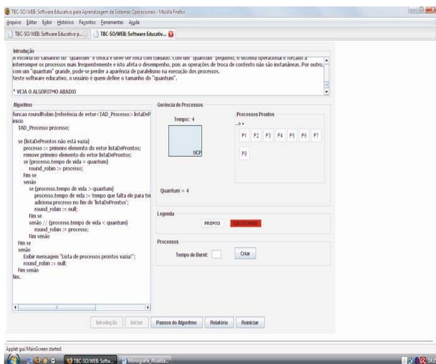
Figura 7-17 – Tela de Execução da Política Round-Robin
