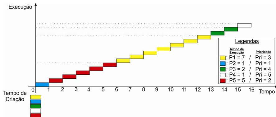
Figura 4-5 – Exemplo de Uso da Política Por Prioridade Não-Preemptiva
