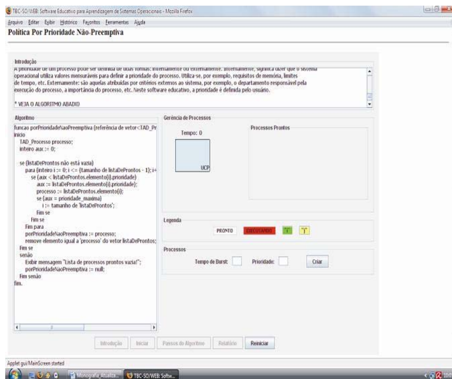
Figura 7-7 – Tela Inicial da Política de Gerência de Processos Por Prioridade Não-Preemptiva
