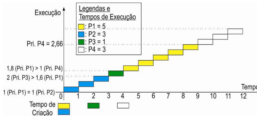
Figura 4-4 – Exemplo de Uso da Política HRRN
