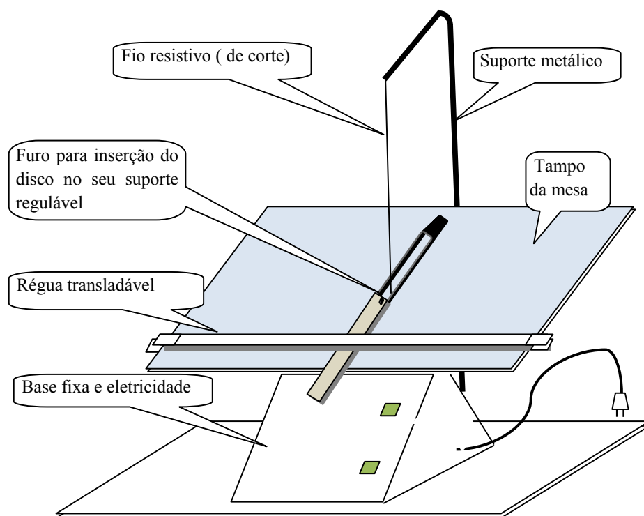
Desenho 1 Máquina para produzir sólidos em isopor
