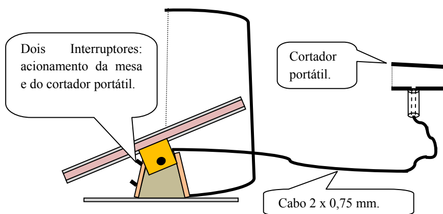
Desenho 21 O cortador portátil e sua instalação, independente do funcionamento da mesa principal
