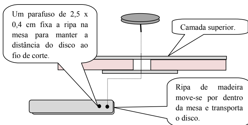
Desenho 9 A construção do tampo com vão por onde corre a ripa de inserção do disco
