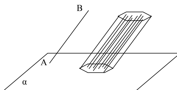
Desenho 28 Ilustração de uma definição de prisma
