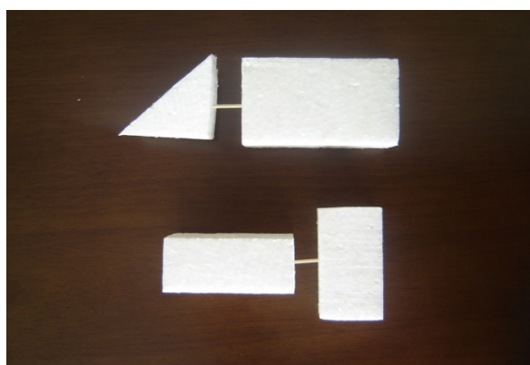
Figura 22 Unindo prismas com palitos de dentes. Com a união das peças observamos que os sólidos obtidos (figura 23) são homeomorfos à esfera
