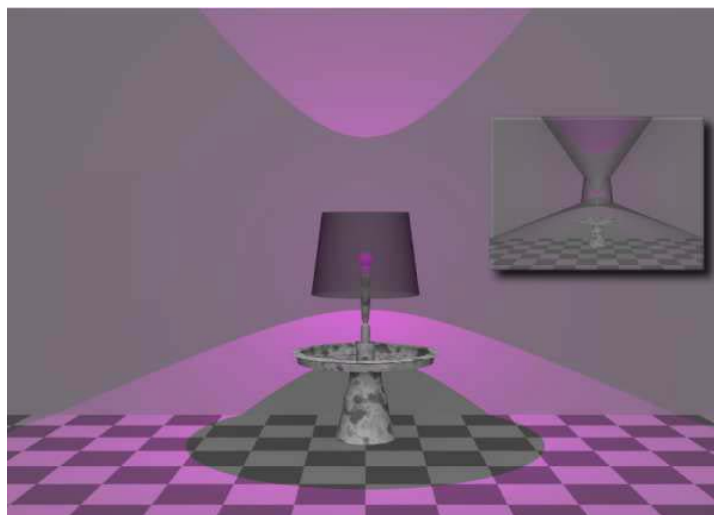
Figura 35 Cones de luz intersectando uma parede podem formar hipérboles variadas
