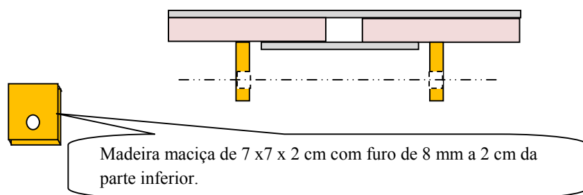
Desenho 11 Suportes fixados ao tampo e que se conectarão à base por meio de dois
