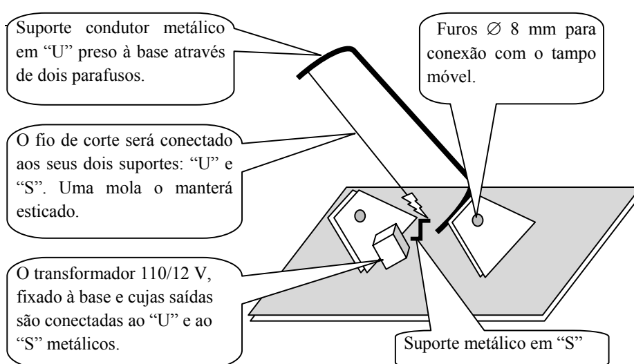
Desenho 3 A base da máquina
