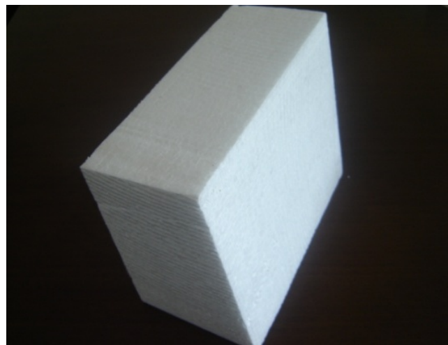
Figura 15 Um prisma quadrangular reto em isopor
