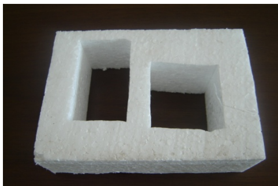
Figura 29 Um sólido com dois furos: Um prisma retangular foi atravessado por outros dois prismas retangulares. Sólido homeomorfo ao bitoro, não é um poliedro
