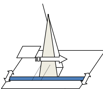
Desenho 26 Geração de uma pirâmide quadrada
