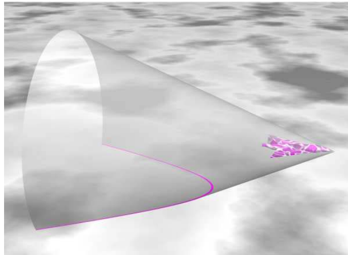
Figura 34 As ondas de choque de um jato supersônico intersectando a superfície do planeta em hipérboles
