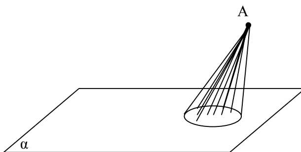
Desenho 31 A definição de cone
