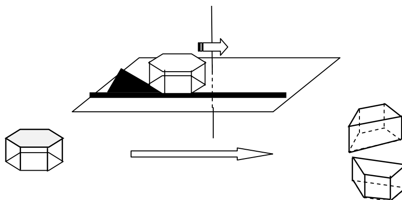
Desenho 35 Na figura, um prisma hexagonal ( F = 8 , A = 18 e V = 12 ), ao ser seccionado por um plano que contém duas de suas arestas laterais opostas, é transformado em dois prismas iguais cujas bases são trapézios ( F = 6 , A = 12 e V = 8 )
