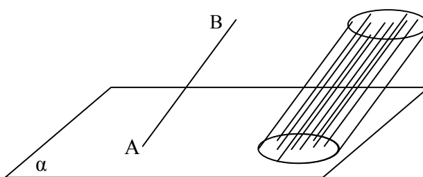
Desenho 30 Ilustrando uma definição de cilindro no Ensino Médio
